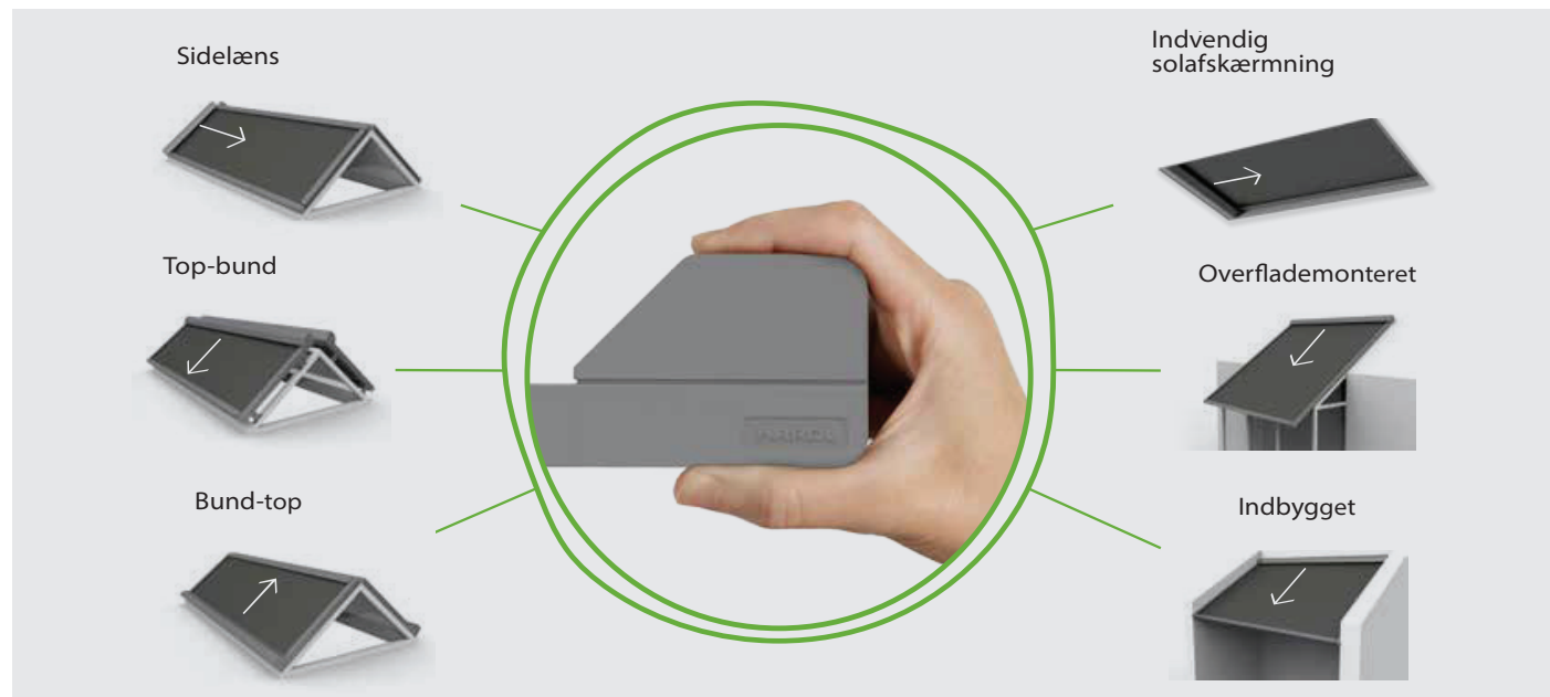
Montagebeslag 1
