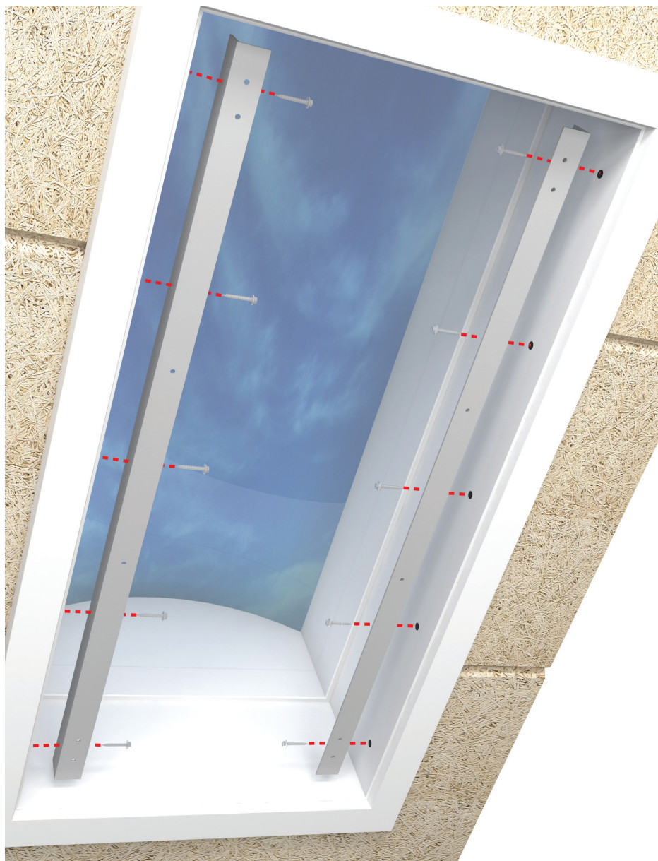
Figur 1: Skru vinklerne A fast til lysningen.
